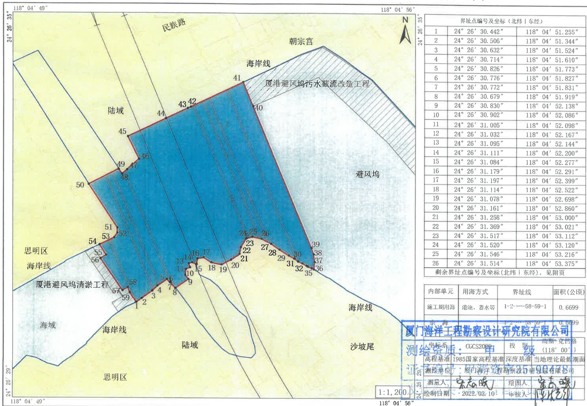
轨道交通3号线南延段工程沙坡尾涉海段(施工期用海)宗海界址图
