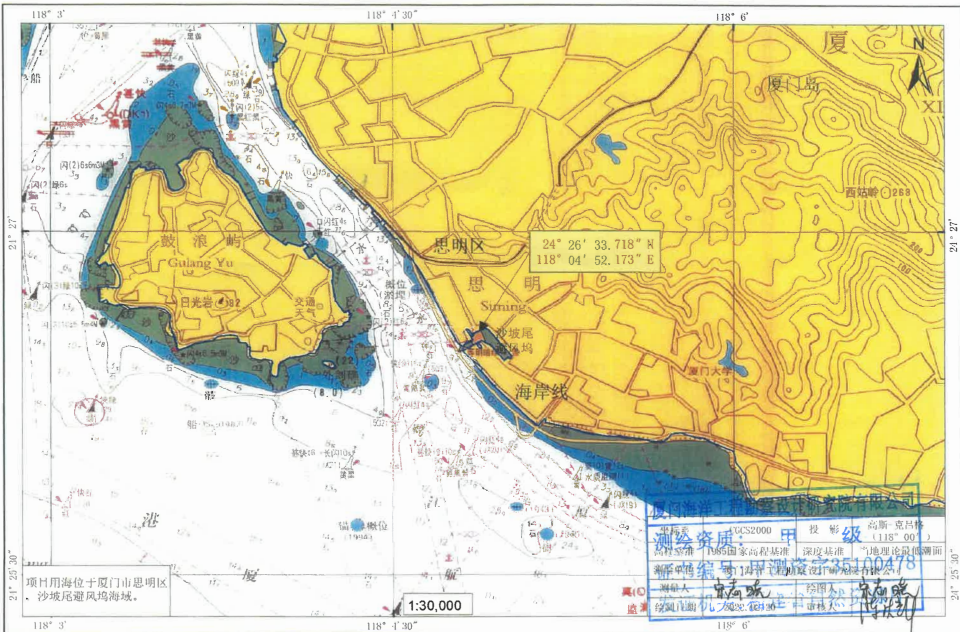
轨道交通3号线南延段工程沙坡尾涉海段宗海位置图
