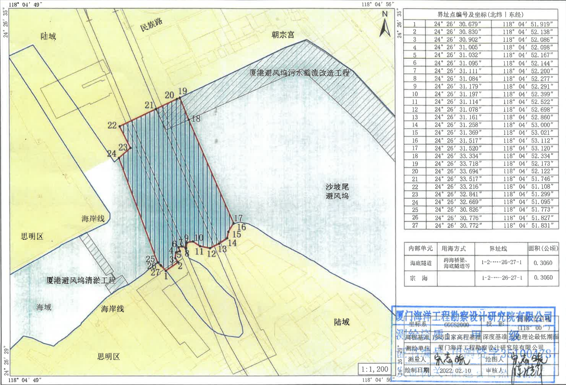
轨道交通3号线南延段工程沙坡尾涉海段(海底隧道)宗海界址图
