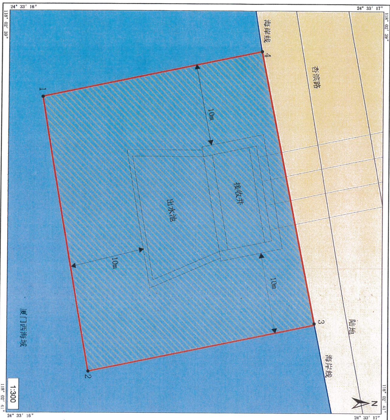
月美池整治工程宗海界址图
